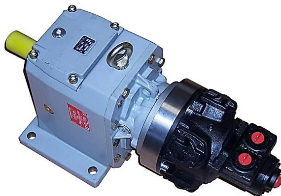
Säteismäntämoottori RM110 hammaspyörävaihteella, RCV
