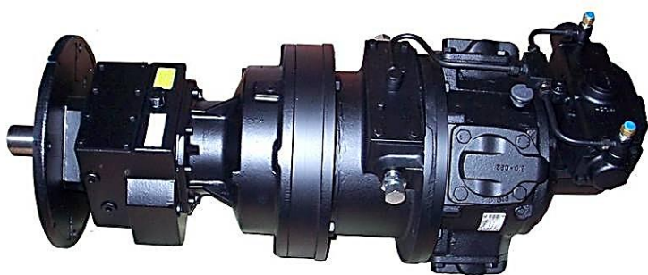
Säteismäntämoottori RM210 jarrulla sekä lieriöhammaspyörävaihteella
