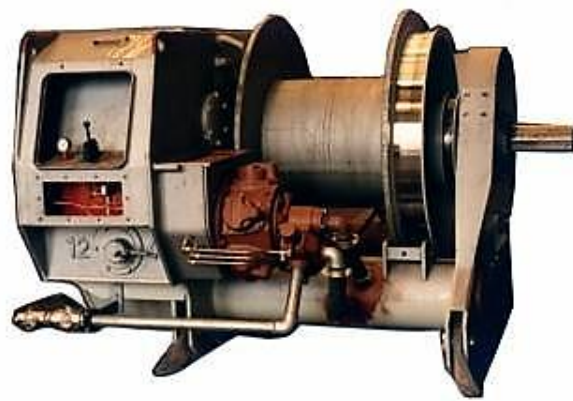
Säteismäntämoottori RM410 vintturikäytössä
