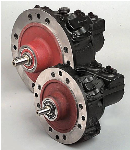
Säteismäntämoottorit RM410 ja RM210
